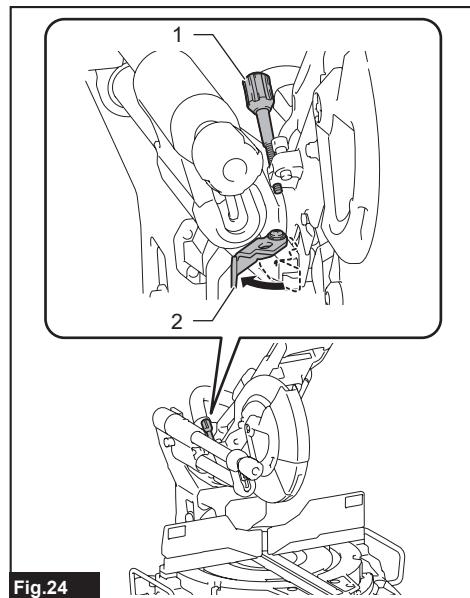
► 1. Vis de réglage 2. Bras de blocage
