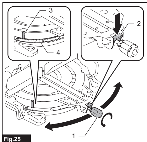
Fig. 25 ► 1. Grip 2. Lock lever 3. Pointer 4. Miter angle scale
